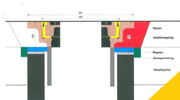
Flydende karm monteret med 30 mm. overhøjde for slidlagsudlægning
